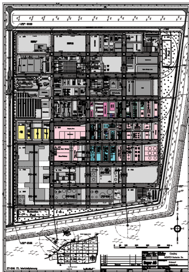
Генеральный план площадки в Каоджинге, КНР
