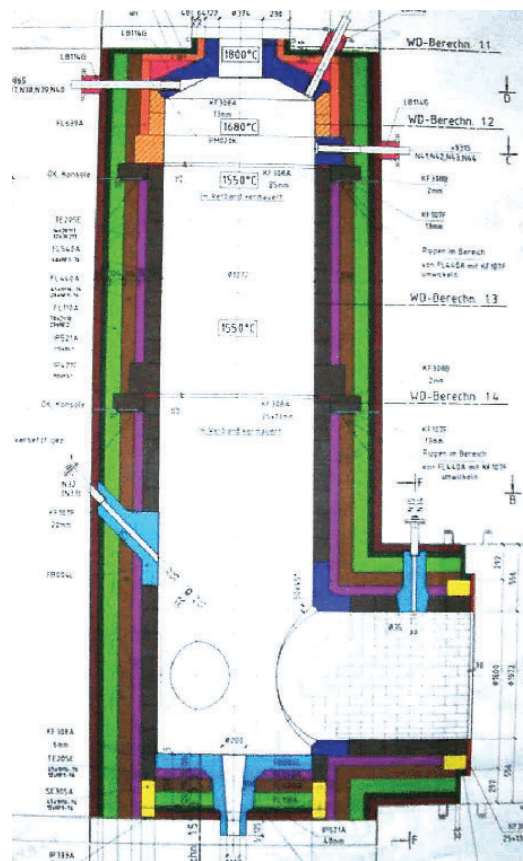
Zeichnungsausschnitt einer feuerfest ausgekleideten Brennkammer (Innentemperaturen 1550 bis 1800 °C)
