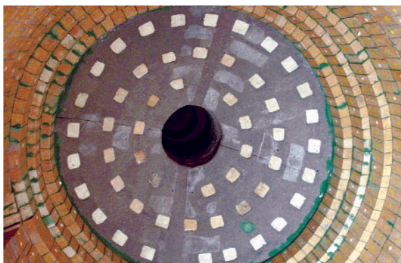
Ausmauerung einer Brennkammerdecke
